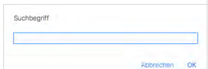
Abb. 6.2 EPG-Suchmaske
