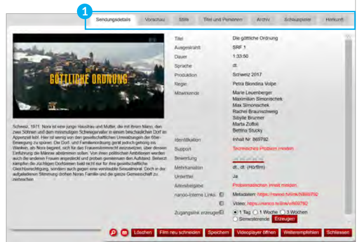
Abb. 7.1 Fenster Sendungsdetails
