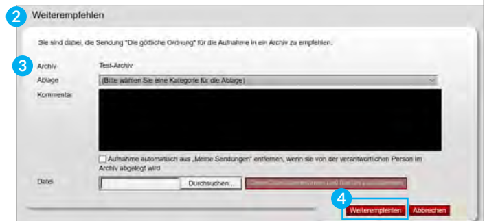
Abb. 8.3 Sendungen weiterempfehlen
