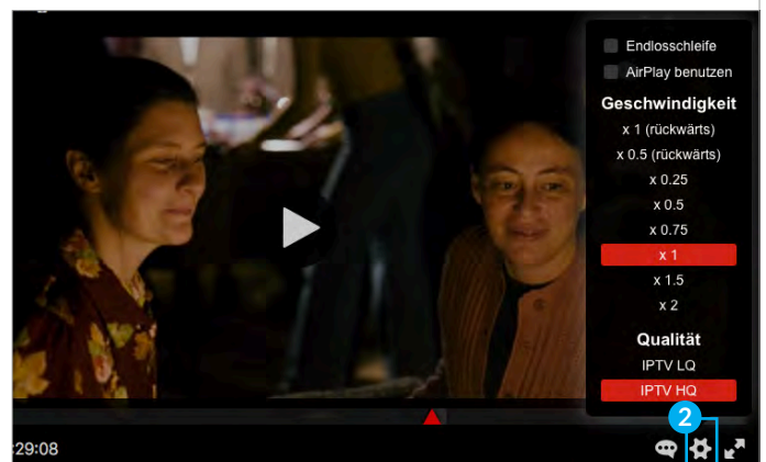
Abb. 9.5 Zusatzfunktionen
